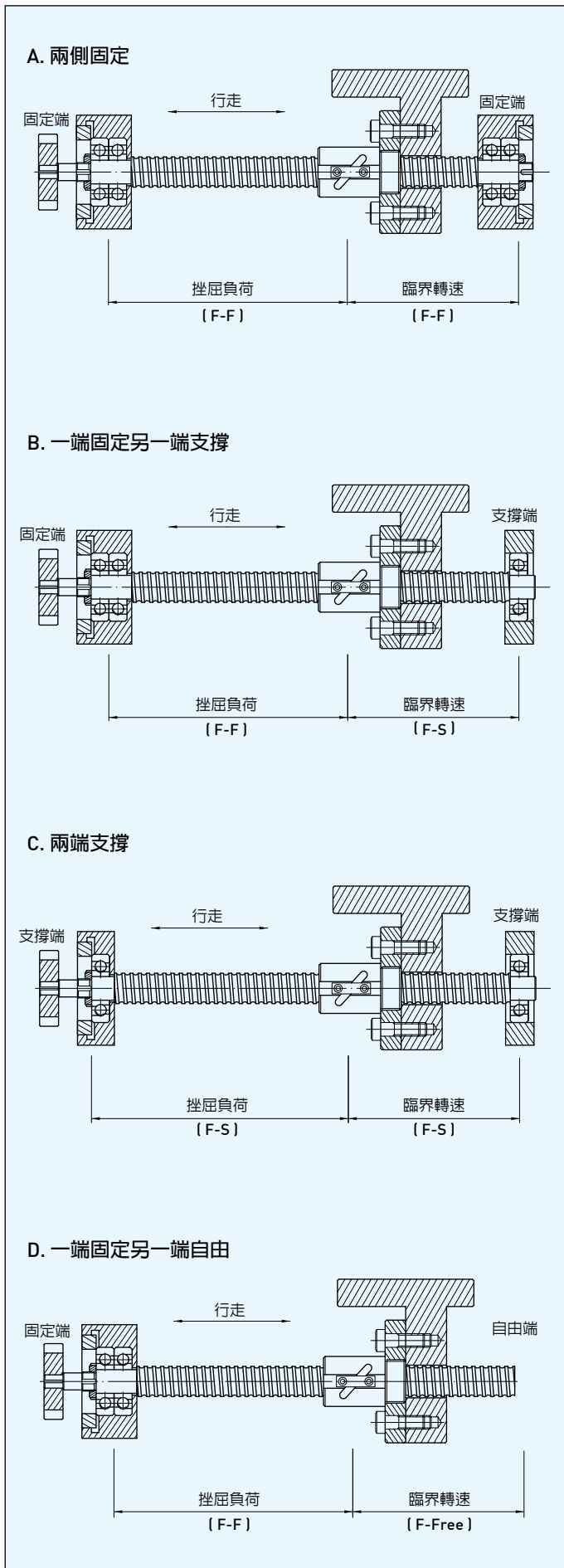
圖3.10 滾珠螺桿安裝實例
