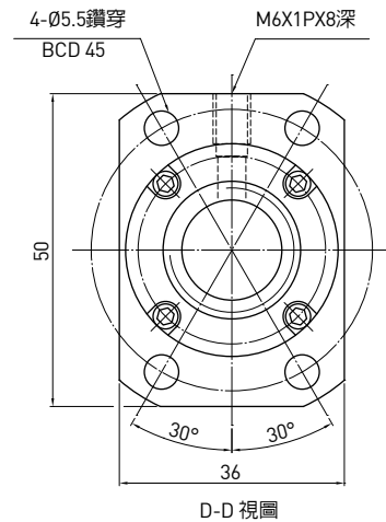
D-D 視圖
