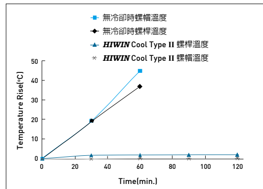
圖 8.9 高速運轉下Cool type II 滾珠螺桿的溫升比較
