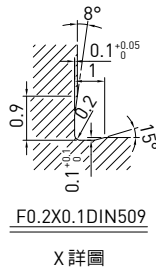
X 詳圖
