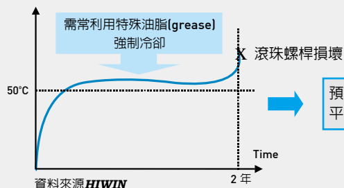
圖8.11 一般射出用滾珠螺桿平均壽命圖
