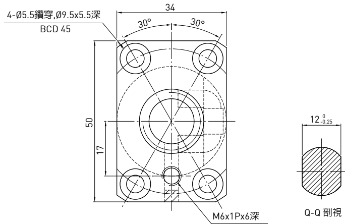
D-D 視圖
