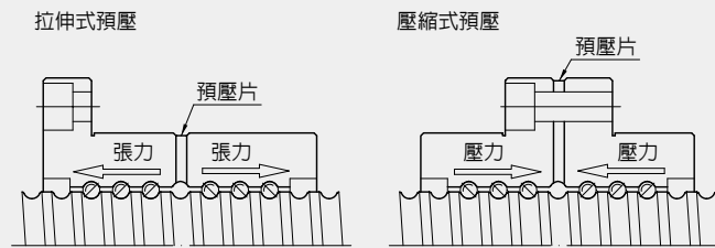
圖4.17 以預壓片尺寸調整預壓方式
