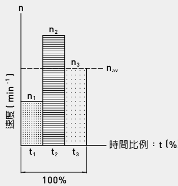
圖 4.22 等效速度
