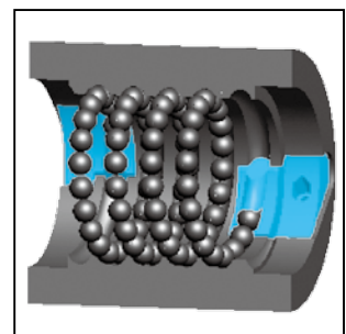
圖3.9 Super S 迴流方式
