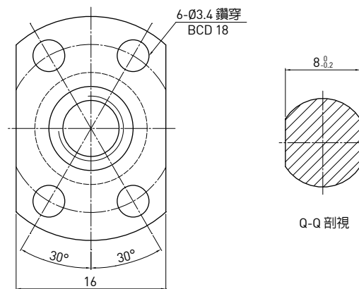
D-D 視圖
