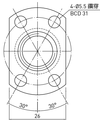
D-D 視圖
