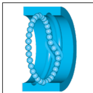
圖3.7 內循環迴流方式
