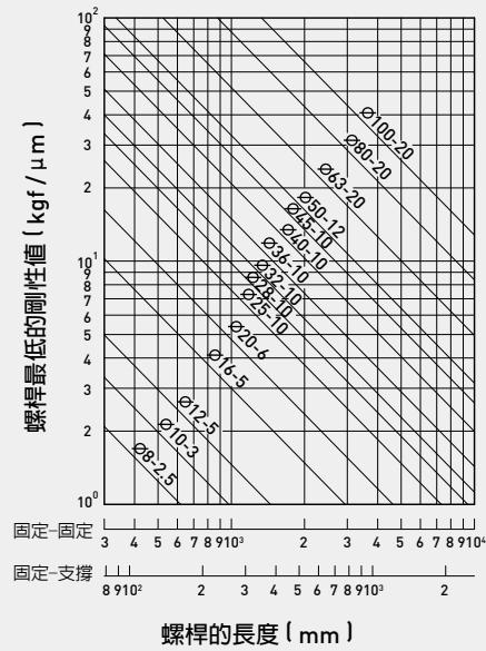
圖 4.29 螺桿剛性表
