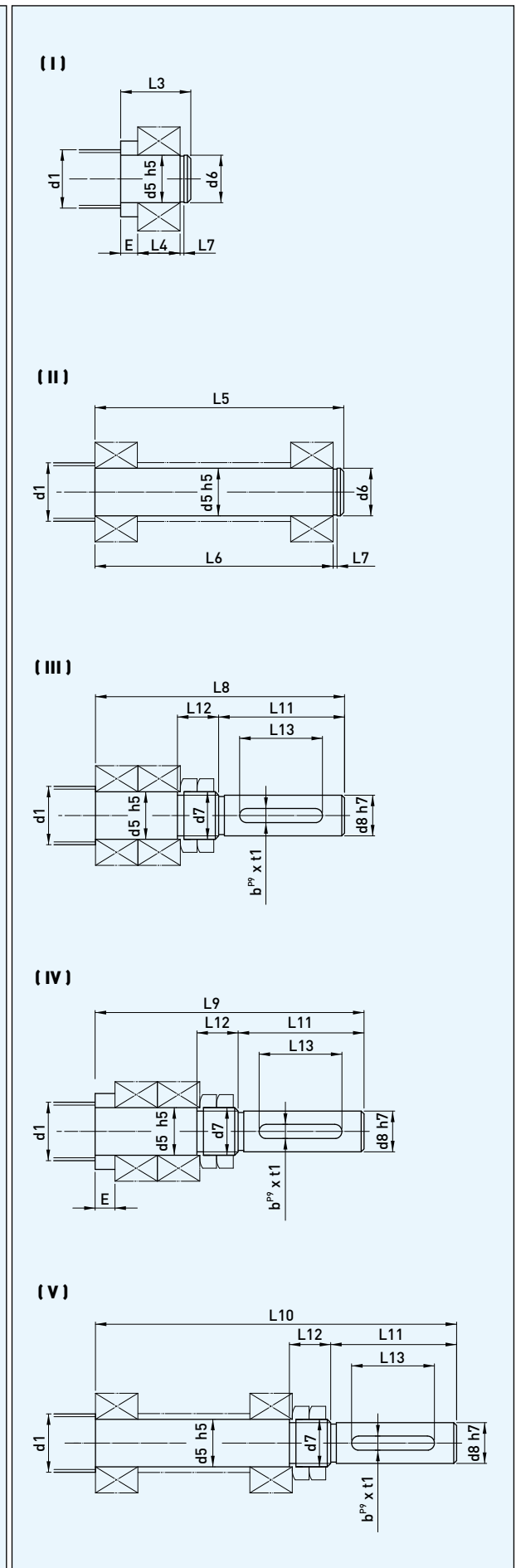
圖3.11 螺桿肩部型式
