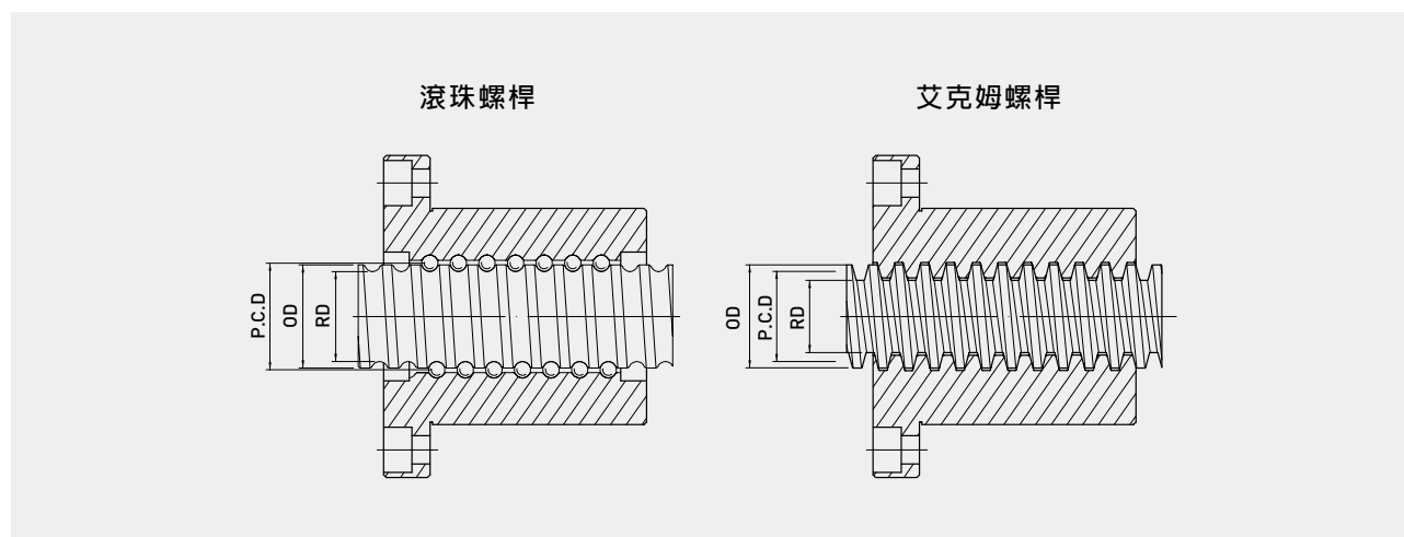
圖2.1 滾珠螺桿與艾克姆螺桿的比較
