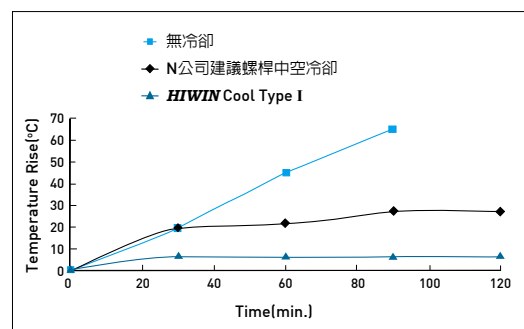
圖8.3 高速運轉下螺桿中空冷卻時，滾珠螺桿的溫升比較
