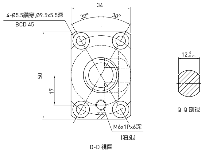
D-D 視圖
