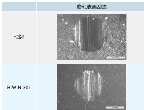
在不同潤滑脂潤滑情況下之鋼球磨耗金相圖
