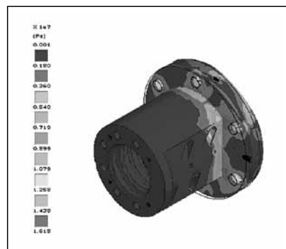
圖8.10 Cool Type滾珠螺桿的有限元素分析
