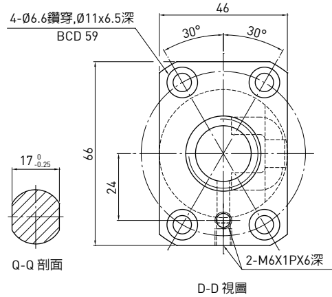
D-D 視圖
