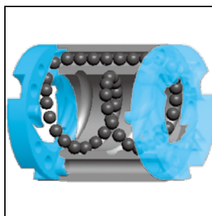
圖3.8 端蓋迴流方式
