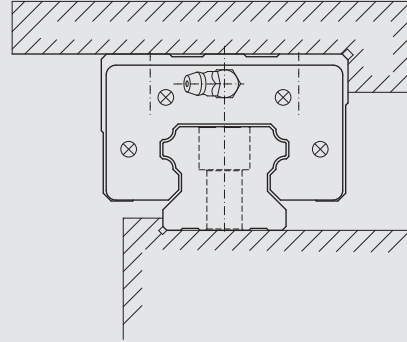
单支导轨有承靠面配置
