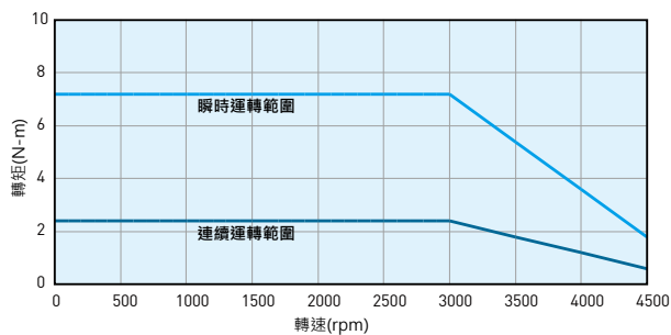
HIWIN FRMS 750W 轉矩-轉速 曲線
