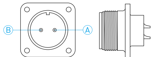
MS3102A14-9P
