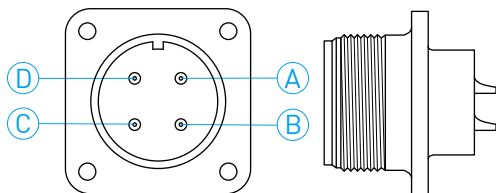
MS3102A18-10P
