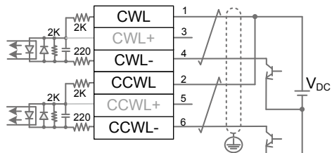
(2) PLC沒有內建電阻之建議配線(使用24V之電源供應)
