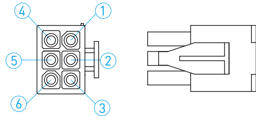
AMP-172168-1(含煞車)
